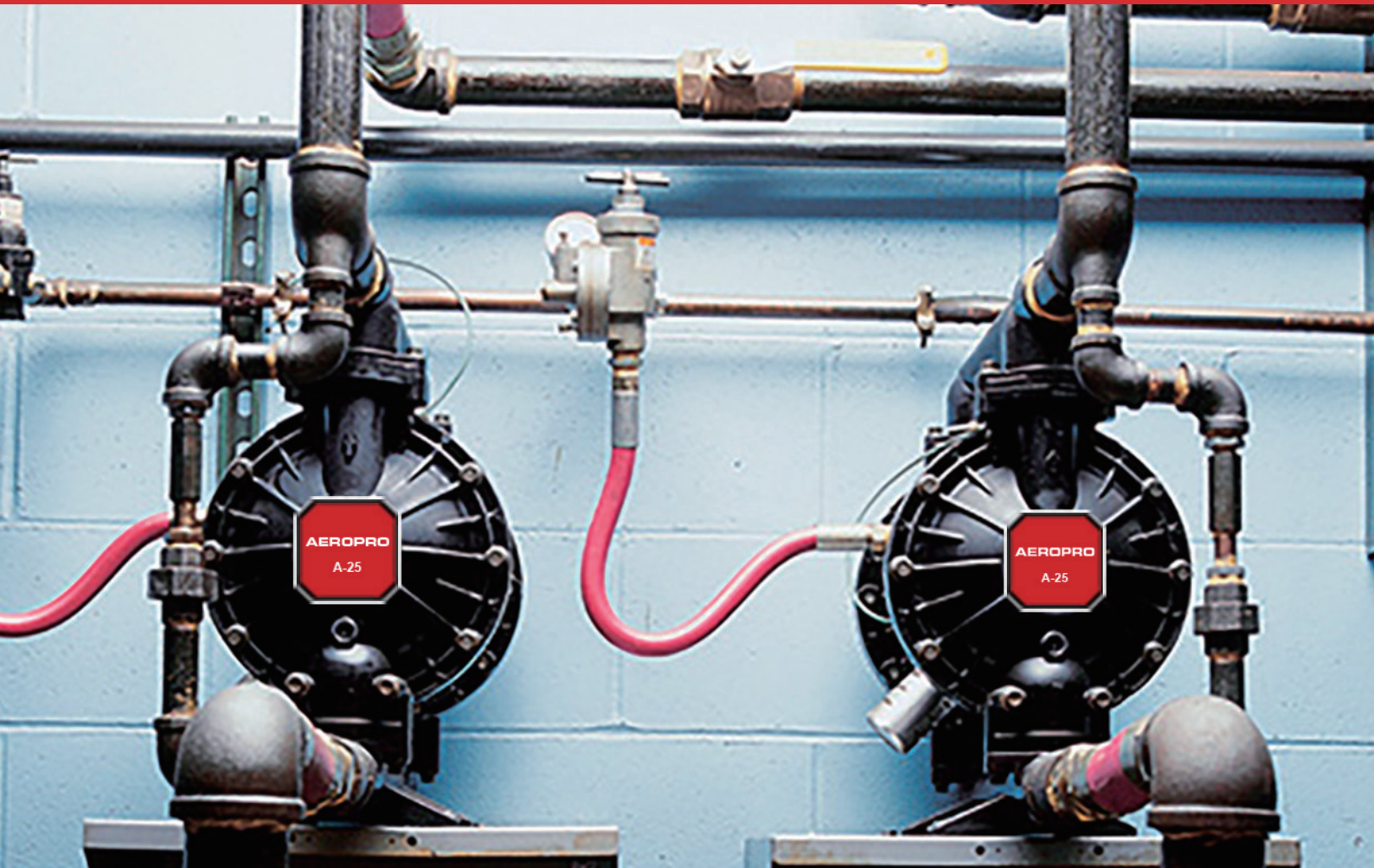
A25 Air Powerd Diaphragm Pump
